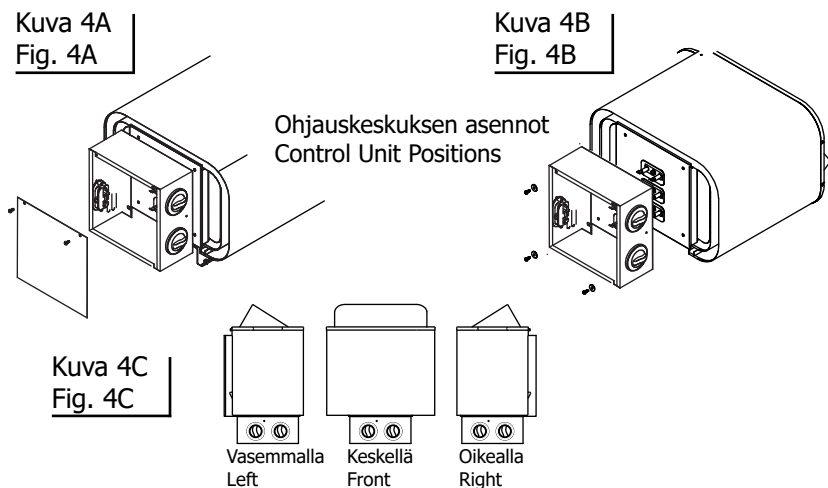
Kuva 4 | Ohjausyksikön avaaminen Fig. 4 | Opening of the Control Unit
