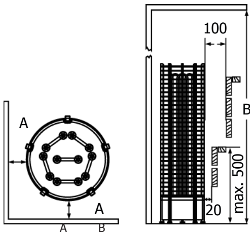
Abb. 2 | Mindest Sicherheitsabstände (mm) Fig. 2 | Minimum Safety Distances (mm)
